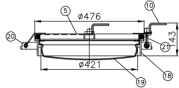
Manhole(M/H)부 상세(1/5)
