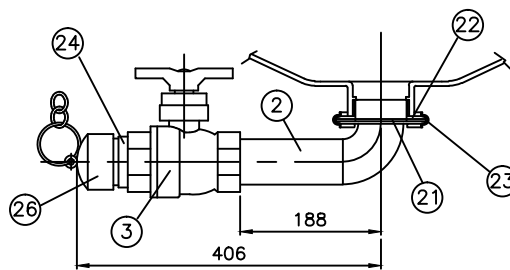
배출관부 상세(1/7.5)
