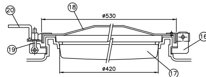
Manhole(M/H)부 상세(1/5)
